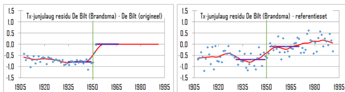
Figuur 34 Links: de door het KNMI toegepaste breukcorrectie op de gemiddelde Tx van juni, juli en augustus. De toegepaste correctie bedraagt gemiddeld -0,8 \pm 0,03 ^{\circ}\text{C} in het interval 1931-1970. Rechts: gevolg van deze breukcorrectie. Het niveauverschil tussen de paarse horizontale lijnen is 0,58 \pm 0,15 ^{\circ}\text{C} .
