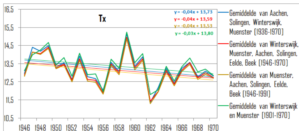
Figuur 43 Gemiddelde T_x (°C) van vier ensembles.
