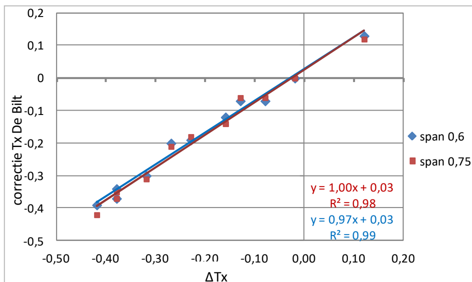
Figuur 38 Relatie tussen jaargemiddelde \Delta T_x (°C) en de gemiddelde Tx correctie De Bilt voor alle vergelijkingsstations (exclusieve percentielen)
