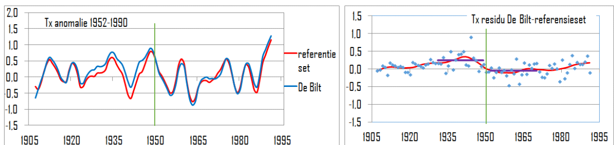
Figuur 29 Links: Tx (°C anomalie van 1952-1990) van De Bilt en de referentieset, Loess-gefilterd met span 8 jaar. Rechts: verschil tussen de jaarlijkse Tx van De Bilt en de jaarlijkse Tx van de referentieset. De rode lijn is een Loess filter met span 15 jaar door de punten. De paarse lijnen stellen de gemiddelde residuen voor in de intervallen 1931-1949 en 1952-1970; het niveauverschil is 0,29 \pm^{15}0,13 °C.
