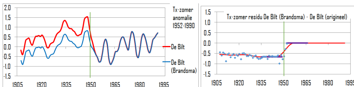
Figuur 32 Links: Tx-zomer ( ^{\circ}\text{C} anomalie van 1952-1990) van De Bilt en de gehomogeniseerde Tx De Bilt, Loess-gefilterd met span 8 jaar. Rechts: verschil tussen Tx-zomer van de door het KNMI gehomogeniseerde De Bilt en de ongehomogeniseerde De Bilt. De paarse lijnen stellen de gemiddelde residuen voor in de intervallen 1931-1949 en 1952-1970; het niveauverschil is 0,67 \pm 0,02 ^{\circ}\text{C} .
