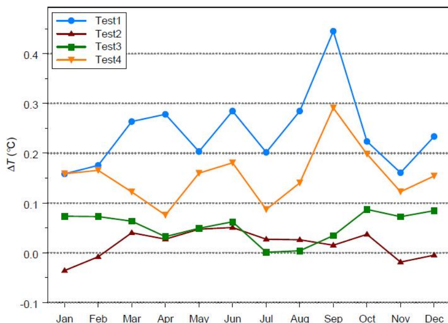
Figuur 12 Verskil tussen de gemiddelde dagelijkse temperatuur per maand van de 4 testlocaties ten opzichte van DB260
