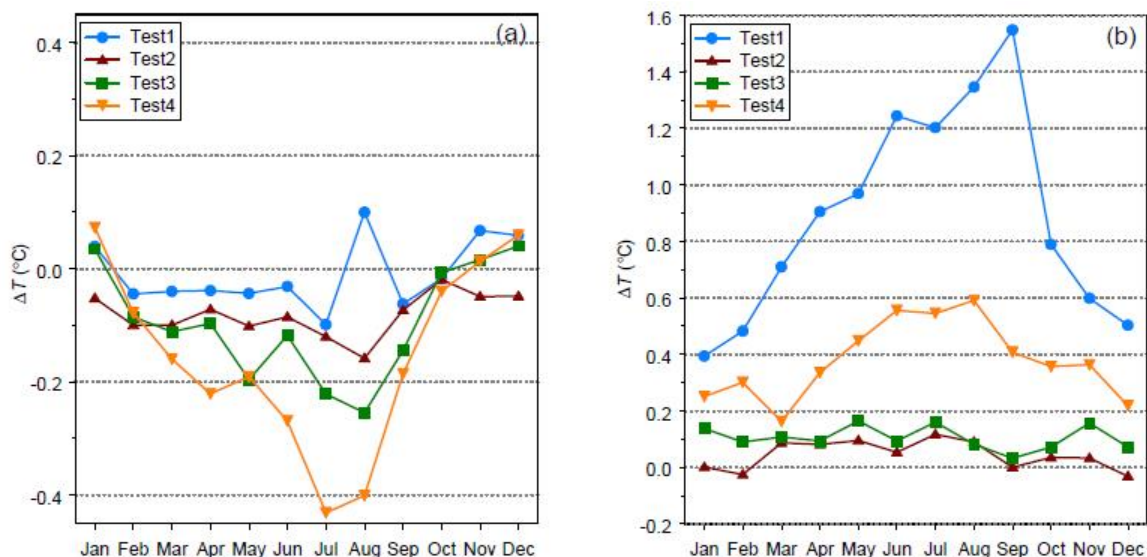
Figuur 13 Verskil tussen de gemiddelde dagelijkse maximum (a) en minimum (b) temperatuur per maand van de 4 testlocaties ten opzichte van DB260
