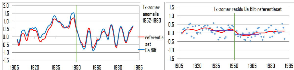
Figuur 31 Links: Tx-zomer ( ^{\circ}\text{C} anomalie van 1952-1990) van De Bilt en de referentieset, Loess-gefilterd met span 8 jaar. Rechts: verschil tussen Tx-zomer van De Bilt en de referentieset. De paarse lijnen stellen de gemiddelde residuen voor in de intervallen 1931-1949 en 1952-1970; het niveauverschil is 0,22 \pm 0,09 ^{\circ}\text{C} .
