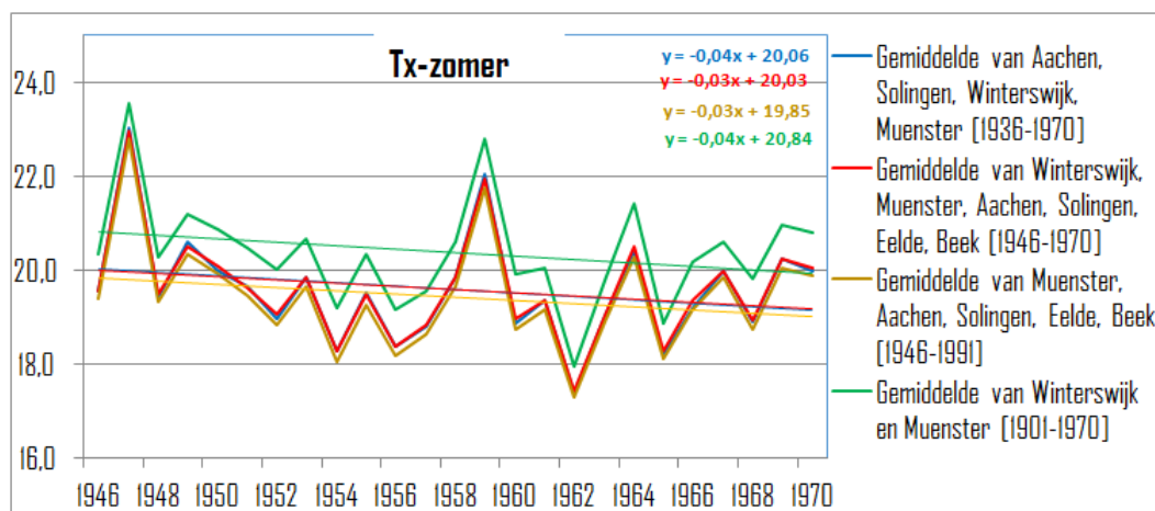
Figuur 45 Gemiddelde Tx-zomer (°C) van vier ensembles.
