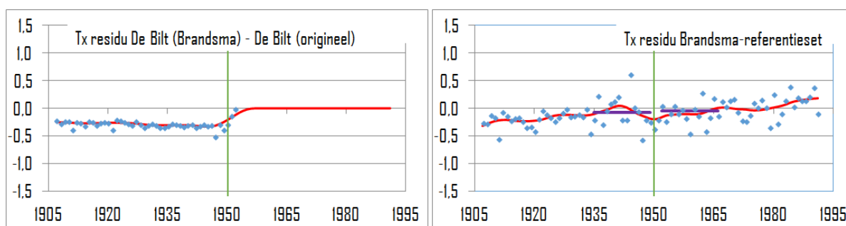
Figuur 30 Links: de breukcorrectie (verschil tussen de jaarlijkse Tx van de door het KNMI gehomogeniseerde De Bilt en de ongehogeniseerde De Bilt). De breukcorrectie is variabel en bedraagt -0,32 \pm 0,01 °C in het interval 1931-1949. Rechts: resultaat van de breukcorrectie op het verschil tussen Tx van de door het KNMI gehomogeniseerde De Bilt en Tx van de referentieset. De rode lijn is een Loess filter met span 15 jaar door de punten. De paarse lijnen stellen de gemiddelde residuen voor in de intervallen 1931-1949 en 1952-1970; het niveauverschil is -0,03 \pm 0,08 °C.
