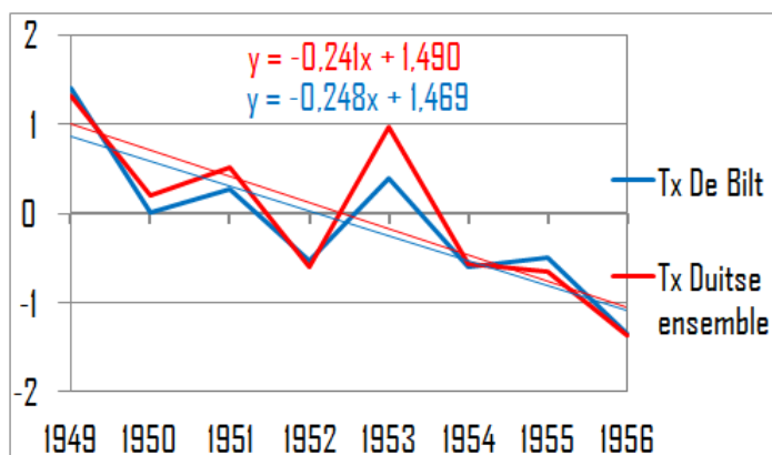
Figuur 23 Tx (°C anomalie van 1952-1990) in het interval van de klimatologische neergang (1949-1956). De Bilt en het Duitse ensemble tonen kwalitatief en kwantitatief dezelfde neergang.
