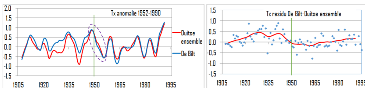
Figuur 22 Links: Tx (°C anomalie van de jaargemiddelde Tx in het interval 1952-1990), Loess-gefilterd met span 8 jaar. De streepjes-ellips markeert de klimatologische neergang en de groene verticale lijn de instrumentele veranderingen rond 1950. Rechts: het verschil (residu) tussen de jaarlijkse Tx in De Bilt en de jaarlijkse Tx van het Duitse ensemble (°C anomalie 1952-1990). De rode lijn is een Loess filter met span 15 jaar door de punten.
