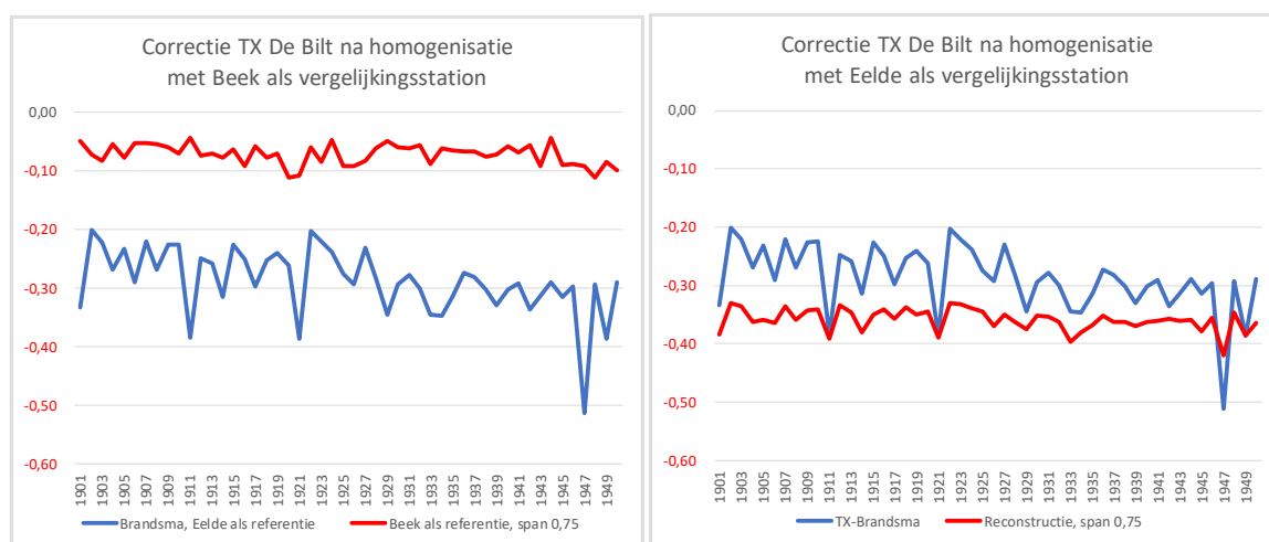
Figuur 37 Effect van de keuze voor Eelde of Beek als vergelijkingsstation op correctie Tx voor De Bilt
