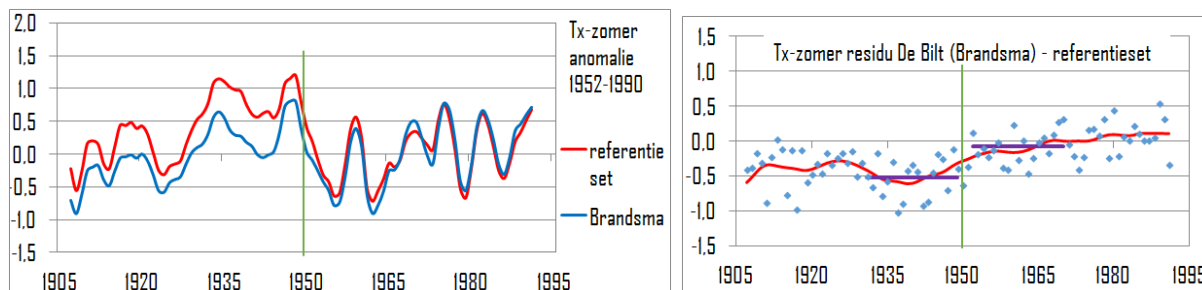
Figuur 33 Links: Tx-zomer ( ^{\circ}\text{C} anomalie van 1952-1990) van de gehomogeniseerde De Bilt en van de referentieset, Loess-gefilterd met span 8 jaar. Rechts: verschil tussen Tx-zomer van de gehomogeniseerde De Bilt en de referentieset. De rode lijn is een Loess filter met span 15 jaar door de punten. Het niveauverschil tussen de paarse horizontale lijnen is 0,45 \pm 0,08 ^{\circ}\text{C} .
