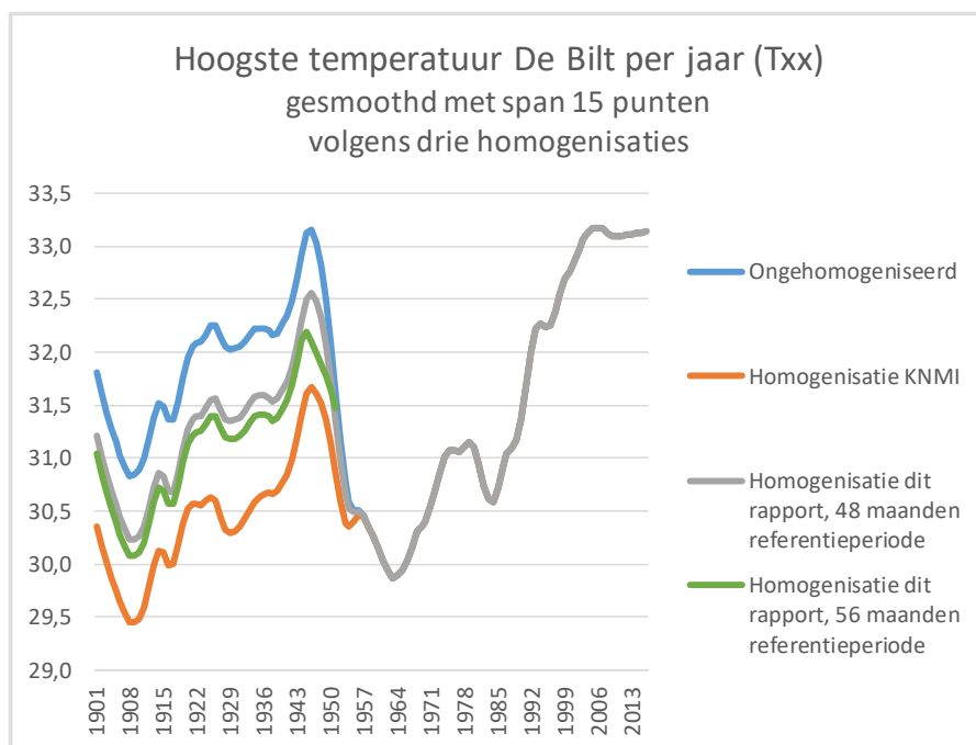
Figuur 21 Trend in de hoogste jaartemperatuur in de Bilt volgens originele metingen KNMI en drie homogenisaties.
