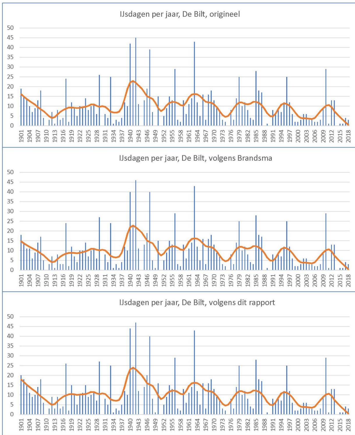
Figuur 56 Aantal ijsdagen dagen per jaar in De Bilt volgens ongehomogeniseerde data, homogenisatie volgens Brandsma en herziene homogenisatie volgens dit rapport. De vloeiende lijn is een Loess-smoothing met een span van 11 punten uit 118 (0,17) om een mogelijke relatie met de zonnecyclus zichtbaar te maken. De homogenisatie volgens dit rapport is evenals die van Brandsma gebaseerd op de data van Eelde (1946-1949 resp. 1952-1955) als vergelijkingsstation. Gebruikte span bij de smoothings 0,75.
