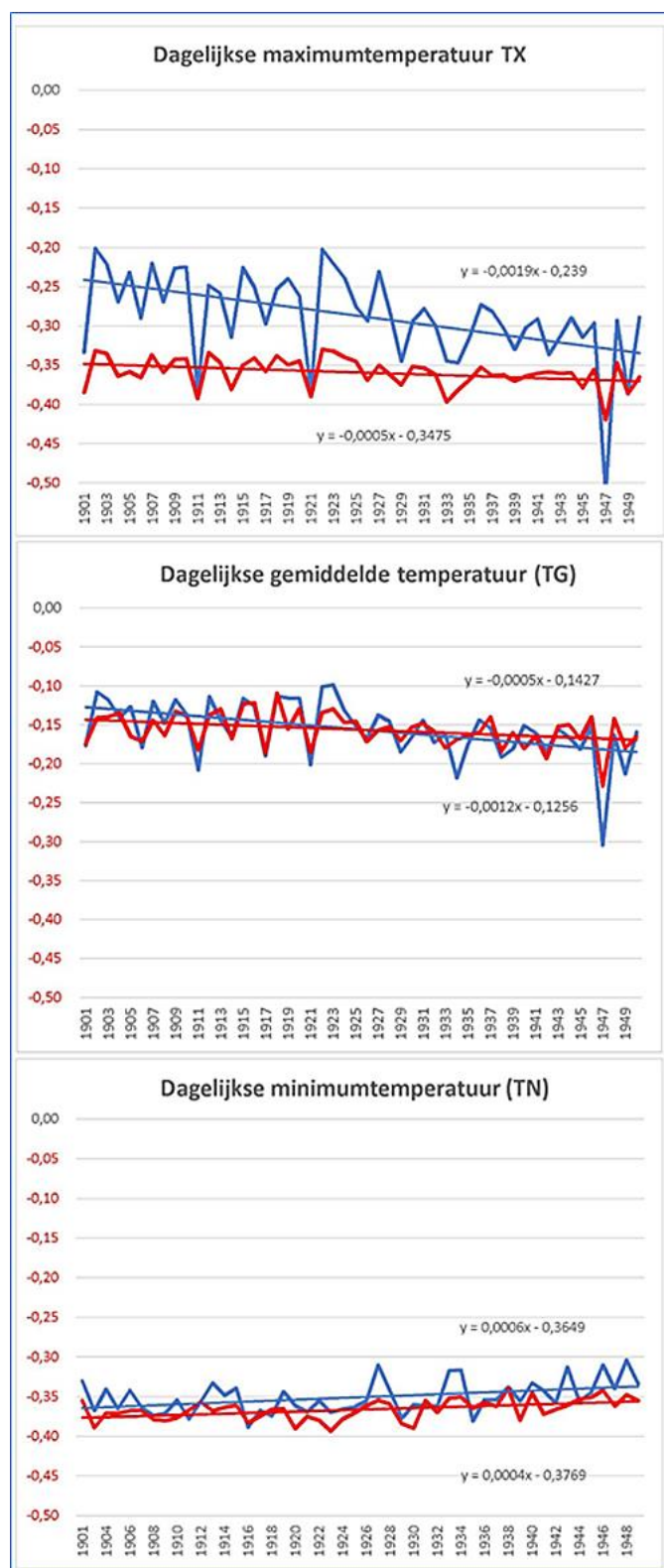
Figuur 18 Gemiddelde correcties per jaar als gevolg van de homogenisatie van Brandsma (blauw) en onze reconstructie van die homogenisatie (rood).
