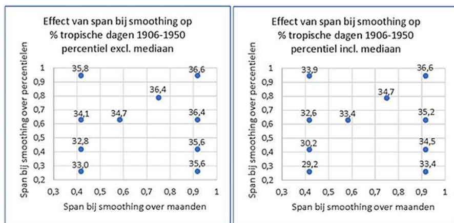
Figuur 17 Effect van span van de smoothing op percentage tropische dagen vóór 1950. Percentielberekening exclusief mediaan (links) en inclusief mediaan (rechts).
